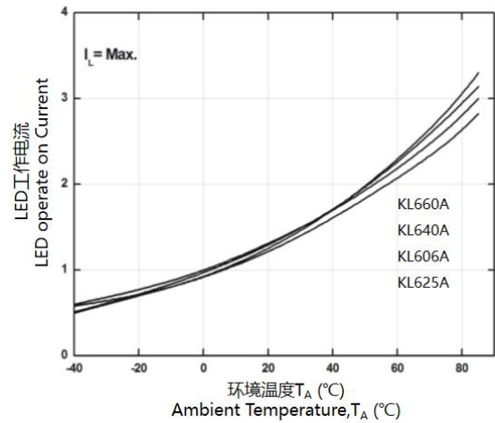
图8. LED下降电压 vs 环境温度的关系
