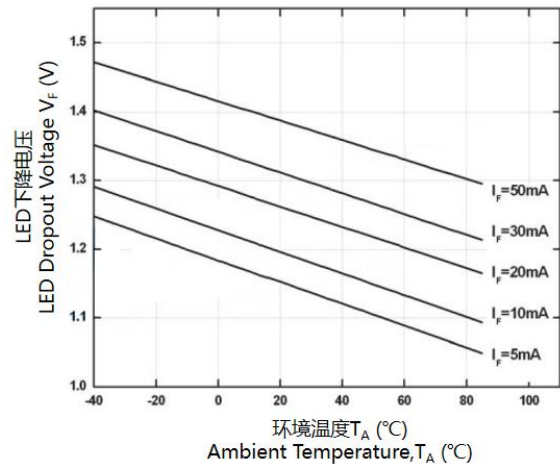
图9-2. 负载电流 vs 负载电压的关系
